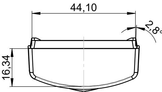
Schnitt C-C
